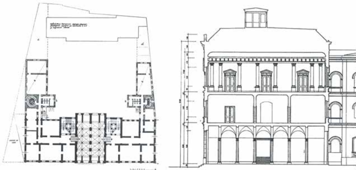
Основа и попречни пресек Здања према Б. Несторовићу
